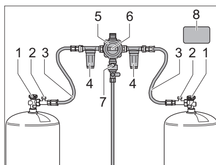
Afb. 82 Caramatic DriveTwo omschakelautomaat
