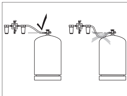
Afb. 84 Aanleggen van de hogedrukslangen
