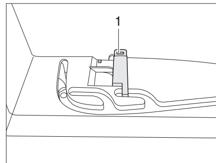
Afb. 46 Vergrendeling ventilatiestand
