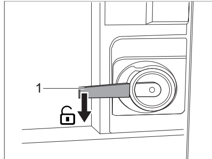
Afb. 22 Deurslot ingangsdeur, binnen, open
