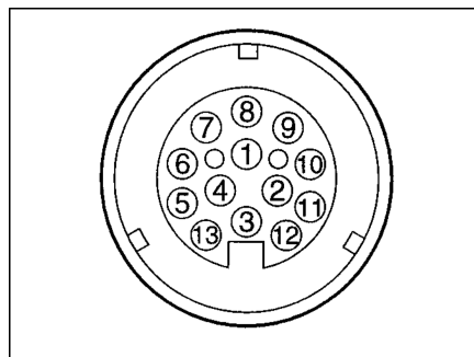
Afb. 98 Aanzicht op de contactdoos van het trekvoertuig (dertienpolig systeem Jaeger conform DIN EN 1648-1)
