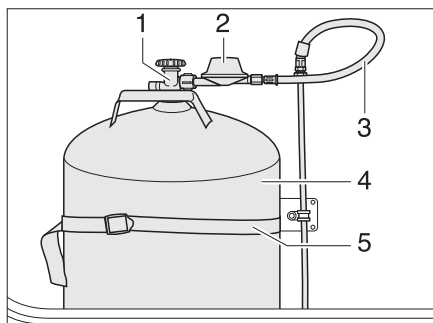
Afb. 79 Gaskast
