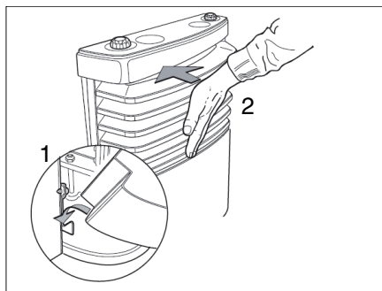
Afb. 107 Breng de behuizing van de verwarming weer aan
