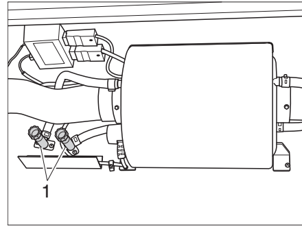
Afb. 124 Locatie van de aftapkranen
