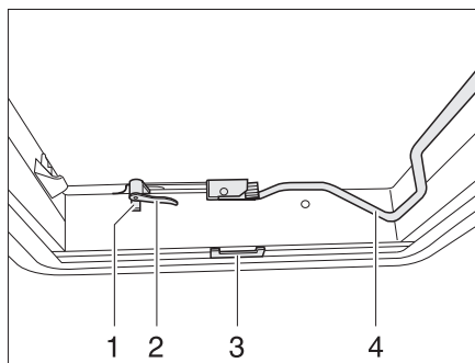
Afb. 47 Heki-dakluik, gesloten
