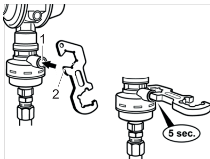
Afb. 86 Crashsensor
