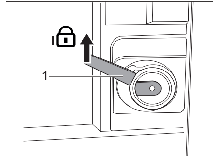
Afb. 23 Deurslot ingangsdeur binnn, vergrendeld, niveau 1
