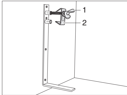
Afb. 162 Reservewielhouder
