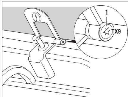
Afb. 126 Scharnieren van de glasafdekking
