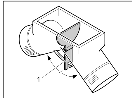
Afb. 111 Circulatieluchtventilator, instelklep in middelste stand
