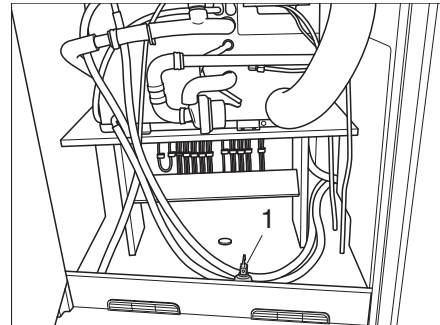
Afb. 121 Locatie van de aftapkranen
