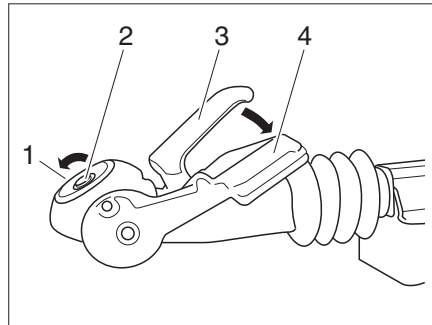
Afb. 1 Veiligheidskoppeling AKS 1300
