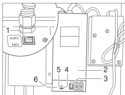
Afb. 117 Transformator met regelapparaat
