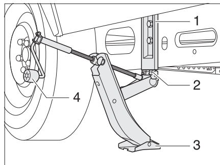
Afb. 189 AL-KO wagenkrik
