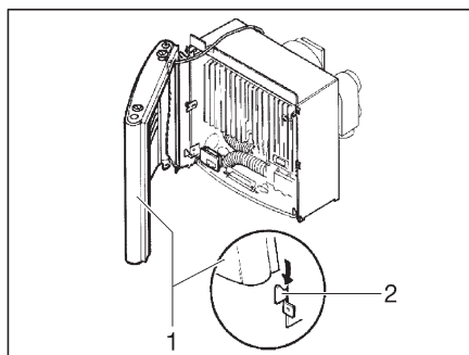
Afb. 109 Behuizing van de verwarming, houderlussen
