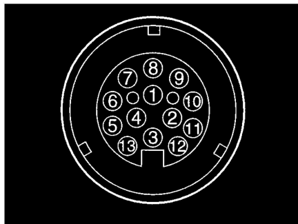
Afb. 102 Zicht op contactdoos trekvoertuig (dertienpolig systeem Jaeger)
