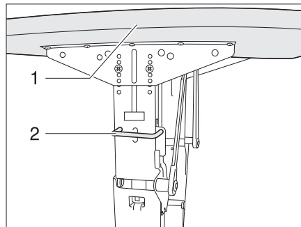
Afb. 60 Vergrendeling zwenktafel met metalen frame
