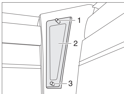
Afb. 181 Indirecte verlichting
