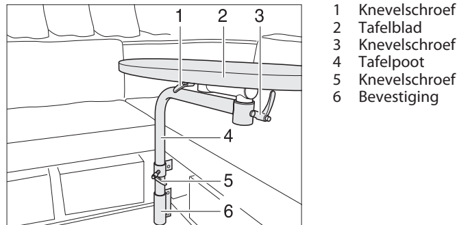
Afb. 61 Zwenktafel
