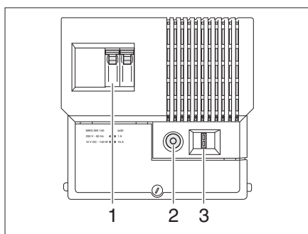
Afb. 89 Stroomvoorzieningsapparaat
