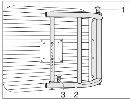
Afb. 65 Zwenkarm voor flatscreen
