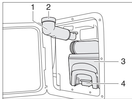
Afb. 159 Thetford-cassette
