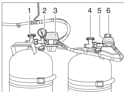
Afb. 87 Duomatic-omschakelinstallatie
