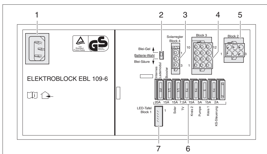
Afb. 92 Elektroblok EBL 109
