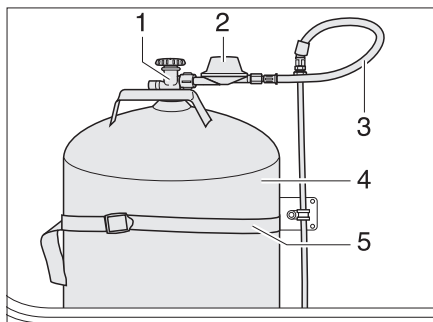
Afb. 84 Gaskast
