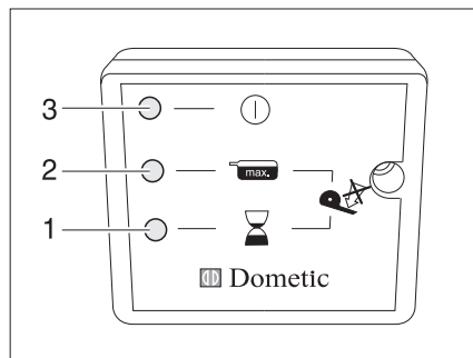
Afb. 162 Paneel vacuüm-toilet
