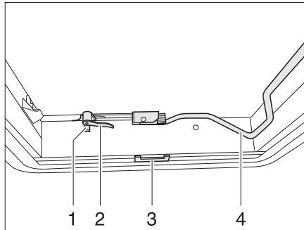
Afb. 51 Heki-dakluik, gesloten
