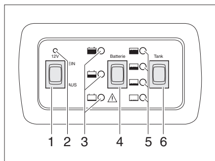
Afb. 93 Paneel LT 109
