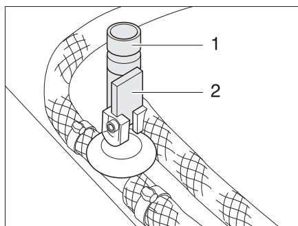
Afb. 127 Aftapkranen voor Truma boiler
