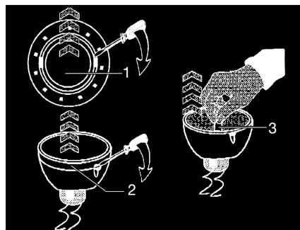
Afb. 178 De halogeengloeilamp verwisselen
