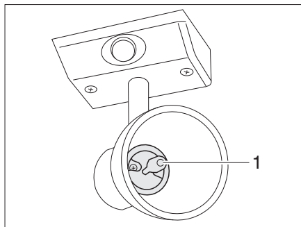
Afb. 176 Halogeenspotlight (met glaskap)
