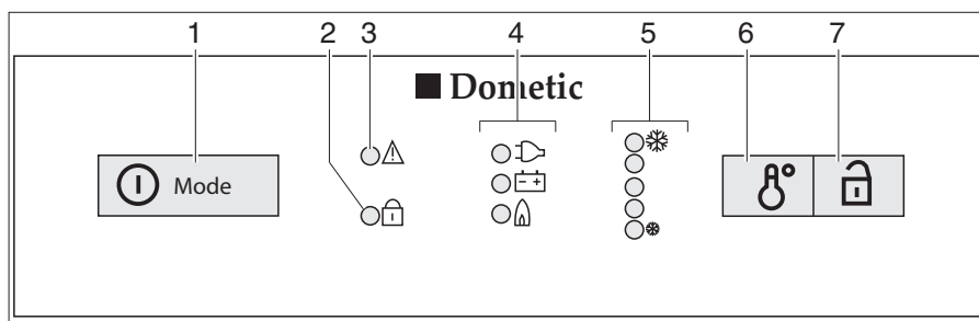
Afb. 140 Bedieningselementen voor de koelkast (Dometic 8-serie met MES)
