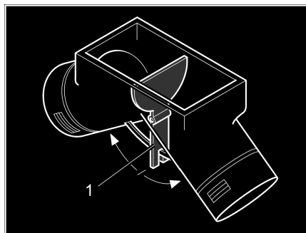
Afb. 113 Circulatieluchtventilator, instelklep in middelste stand
