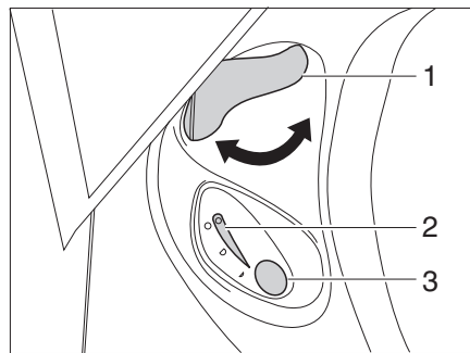
Afb. 160 Bedieningspaneel Thetford-toilet
