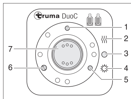
Afb. 148 Bedieningspaneel
