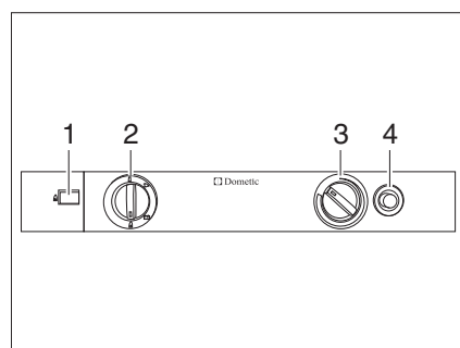
Afb. 200 Bedieningselementen voor de koelkast (Dometic 8-serie)
