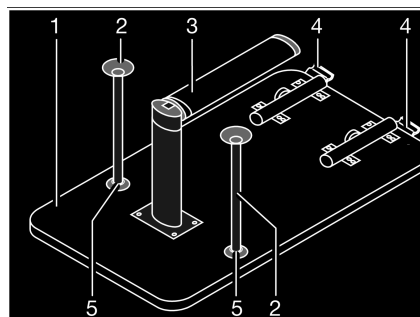
Afb. 72 Bed-onderstel
