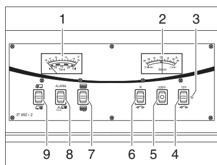
Afb. 151 Paneel IT 992
