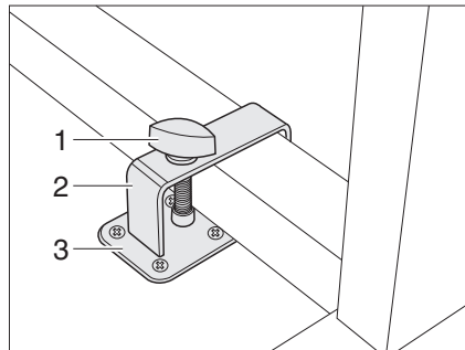
Afb. 76 Vergrendeling zwenktafel met beugel
