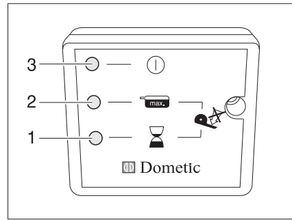
Afb. 243 Paneel vacuüm-toilet
