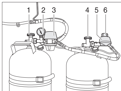
Afb. 145 Duomatic-omschakelinstallatie
