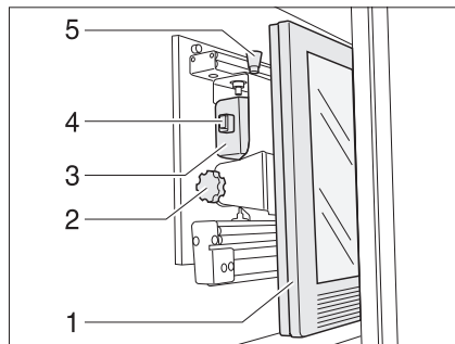
Afb. 83 TV-kast
