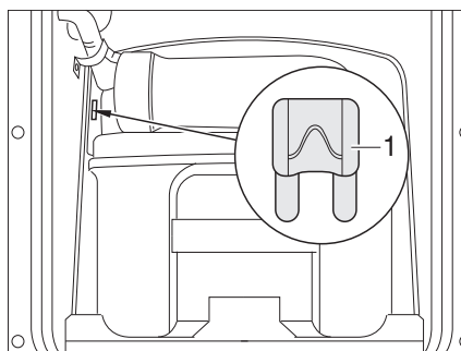
Afb. 158 Zekering van het Thetford-toilet
