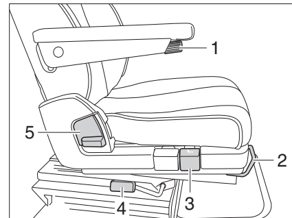
Afb. 70 Bestuurdersstoel en passagiersstoel (ISRI)
