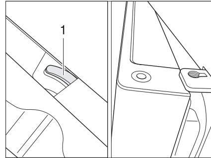
Afb. 207 Koelkastdeur/vriesvakdeur in ventilatiestand (Dometic 7-serie met apart vriesvak)
