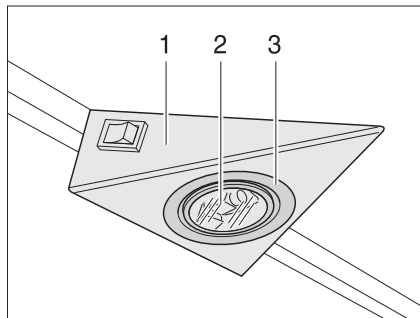
Afb. 259 Halogeen-inbouwlamp
