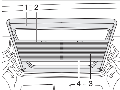
Afb. 56 Dakraam
