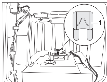
Afb. 159 Zekering van het Thetford-toilet (alternatief)
