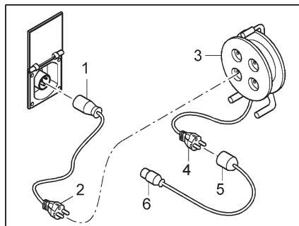
Afb. 153 Aansluitmogelijkheden 230-V-aansluiting
