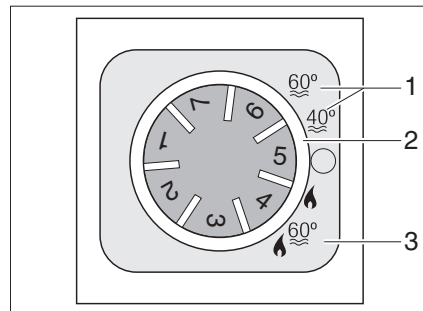
Afb. 182 Bedieningspaneel voor verwarming/boiler
