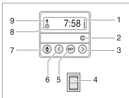
Afb. 174 Bedieningspaneel voor standverwarming
