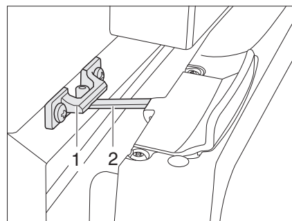
Afb. 213 Koelkastdeur in ventilatiestand (Thetford)
