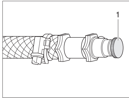
Afb. 252 Ontluchtingsventiel warmwaterverwarming
