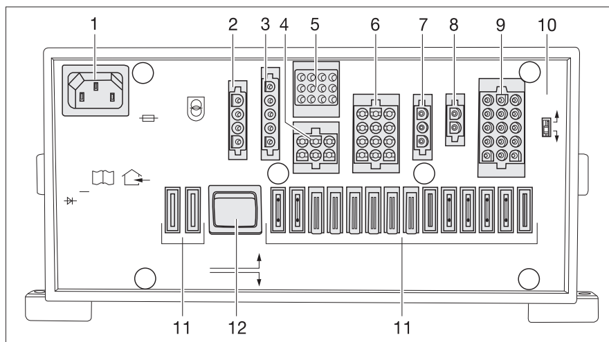
Afb. 149 Elektroblok (EBL 99)
