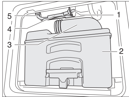
Afb. 249 Afvoerslang watertank toilet
