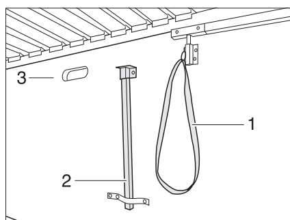
Afb. 97 Steun en ontgrendeling
