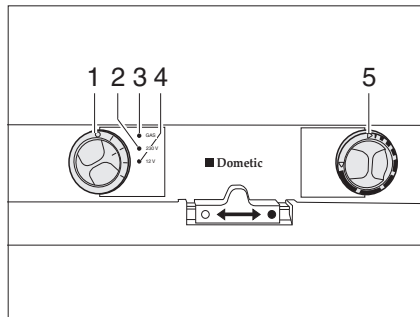
Afb. 198 Bedieningselementen voor de koelkast (Dometic 7-serie)
