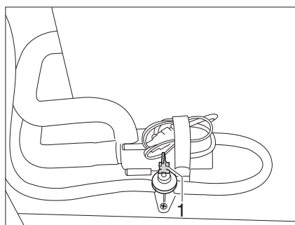
Afb. 225 Aftapkraan
