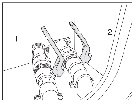
Afb. 216 Aftapkraan in de dubbele bodem
