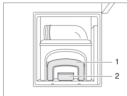
Afb. 247 Toegang fecaliëntank, geopend
