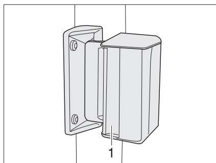
Afb. 48 Schuifraam
