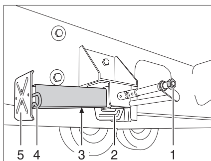
Afb. 30 Hefsteun
