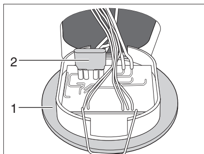
Afb. 161 Zekering van het toilet
