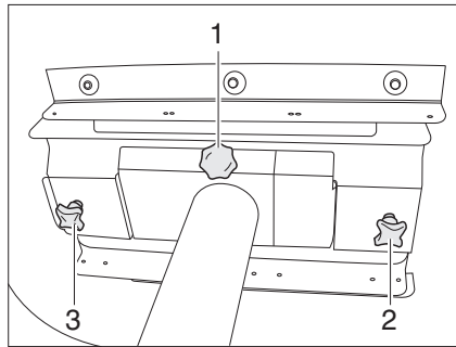
Afb. 80 Vaste tafel (aanzicht van onder)
