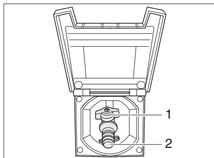
Afb. 144 Externe gasaansluiting, gasafsluitkraan gesloten
