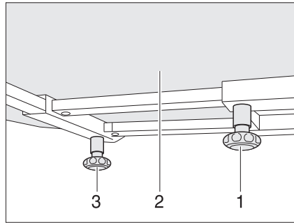
Afb. 78 Vaste tafel
