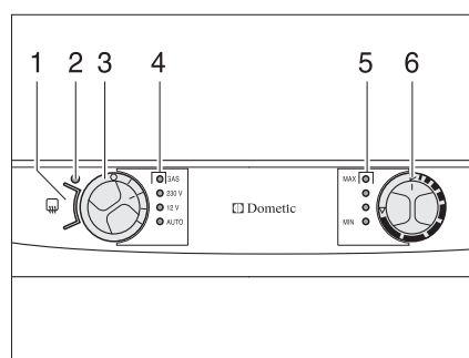
Afb. 199 Bedieningselementen voor de koelkast (Dometic 7-serie met AES en FV)
