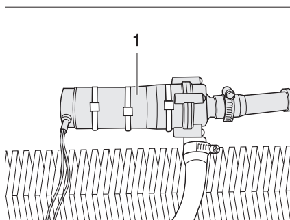
Afb. 171 Extra circulatiepomp
