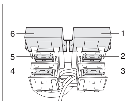
Afb. 156 Zekeringen voor de startaccu
