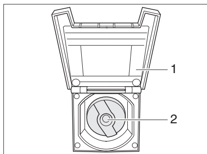
Afb. 215 Afsluitdeksel voor drinkwatervulopening
