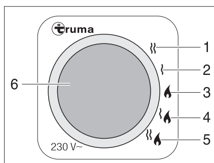
Afb. 184 Energiekeuzeschakelaar voor verwarming/boiler
