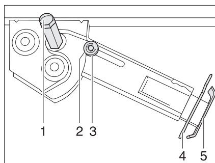
Afb. 31 Hefsteun
