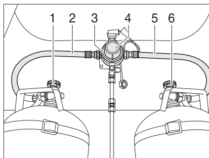
Afb. 147 DuoControl-omschakelinstallatie
