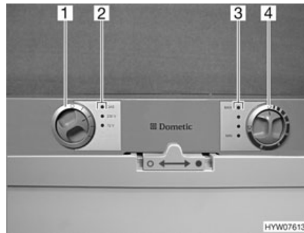
Afb. 150 Bedieningselementen voor de koelkast (Dometic 7-serie met AES)
