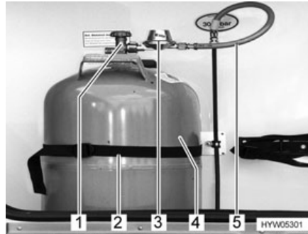
Afb. 94 Gaskast
