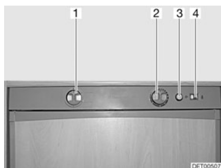
Afb. 148 Bedieningselementen voor de koelkast (Dometic 7-serie met handmatige ontsteking)
