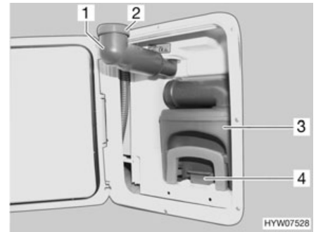
Afb. 168 Thetford-cassette
