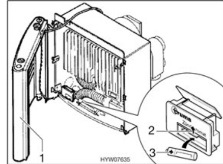
Afb. 118 Verwarming geopend
