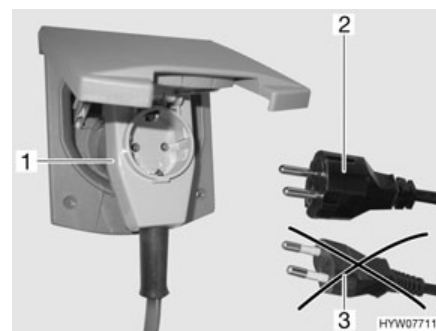
Afb. 106 Aansluiting aan een hoekkoppeling met contactdoos
