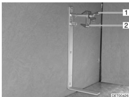
Afb. 199 Reservewielhouder
