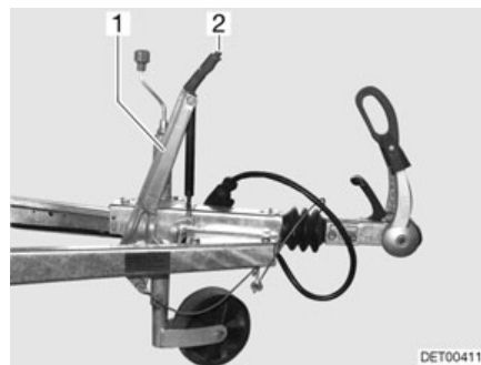
Afb. 15 Handrem
