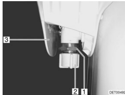
Afb. 176 Ventiel vacuüm-toilet
