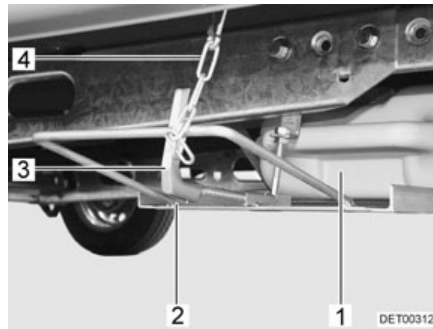
Afb. 162 Afvalwatertank in houder onder het voertuig
