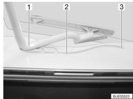
Afb. 50 Heki-dakluik, geleiding
