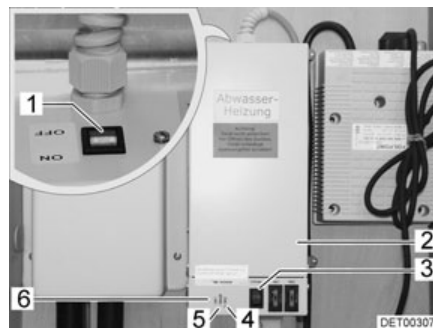
Afb. 128 Transformator met regelapparaat
