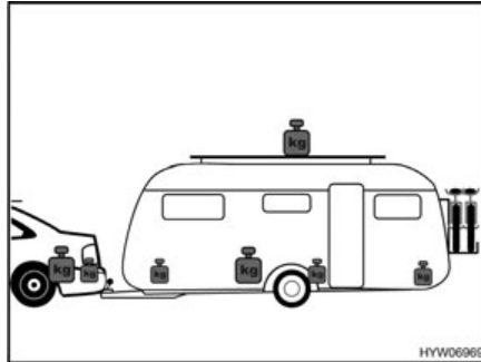
Afb. 3 Verkeerde gewichtsverdeling
