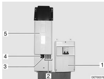
Afb. 100 Stroomvoorzieningsapparaat (type I)
