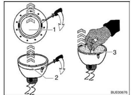
Afb. 187 De halogeengloeilamp verwisselen
