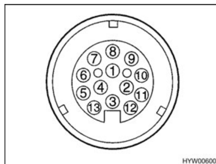
Afb. 112 Zicht op contactdoos trekvoertuig (dertienpolig systeem Jaeger)
