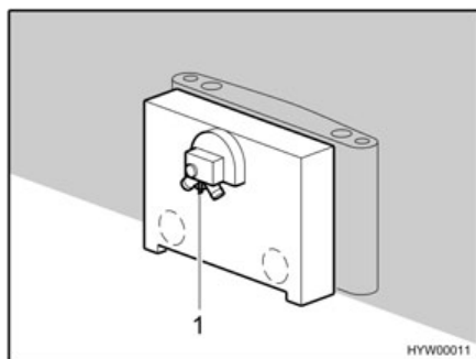
Afb. 122 Circulatieluchtventilator
