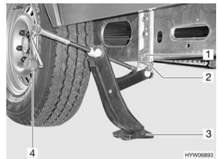
Afb. 198 AL-KO wagenkrik
