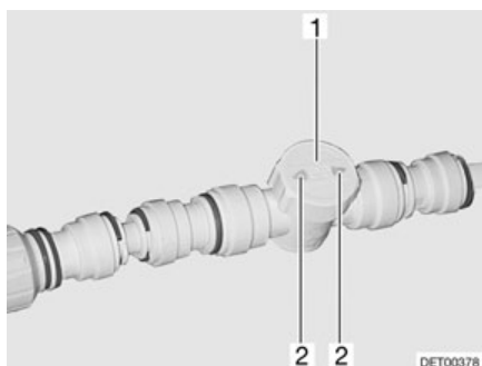
Afb. 130 Regelaar vloerverwarming/verwarming voor afvalwatertank
