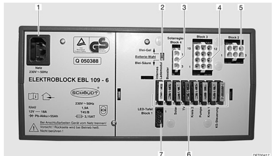
Afb. 102 Elektroblok EBL 109
