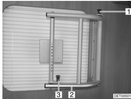
Afb. 68 Zwenkarm voor flatscreen
