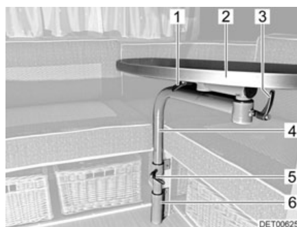
Afb. 64 Zwenktafel
