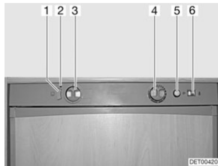
Afb. 149 Bedieningselementen voor de koelkast (Dometic 7-serie met handmatige ontsteking en frameverwarming)
