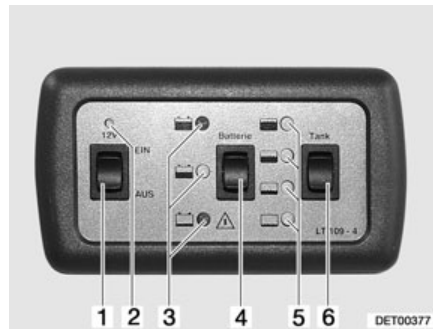
Afb. 103 Paneel LT 109
