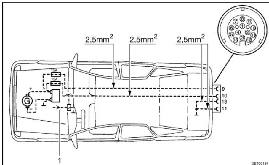
Afb. 113 Trekwagen-installatieschema (autark-pakket)
