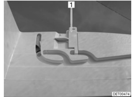
Afb. 52 Vergrendeling ventilatiestand
