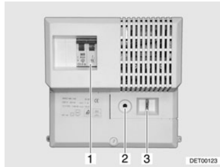
Afb. 99 Stroomvoorzieningsapparaat
