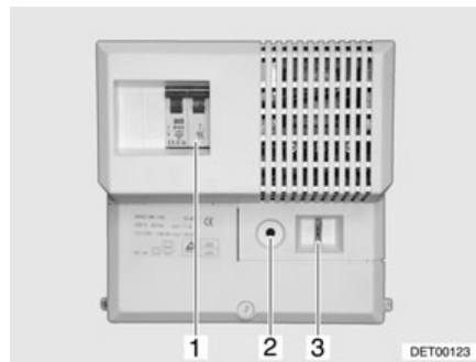
Afb. 110 Beveiligingsautomaat (variant 1)
