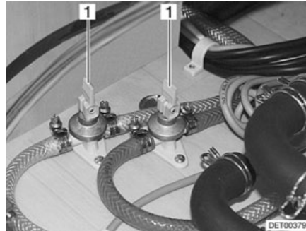
Afb. 136 Aftapkranen
