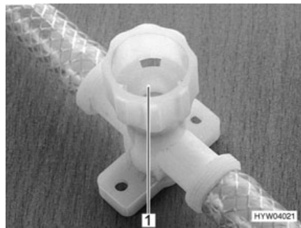
Afb. 139 Aftapkraan voor verwarmingsketel
