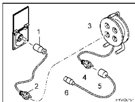
Afb. 105 Aansluitmogelijkheden 230-V-aansluiting
